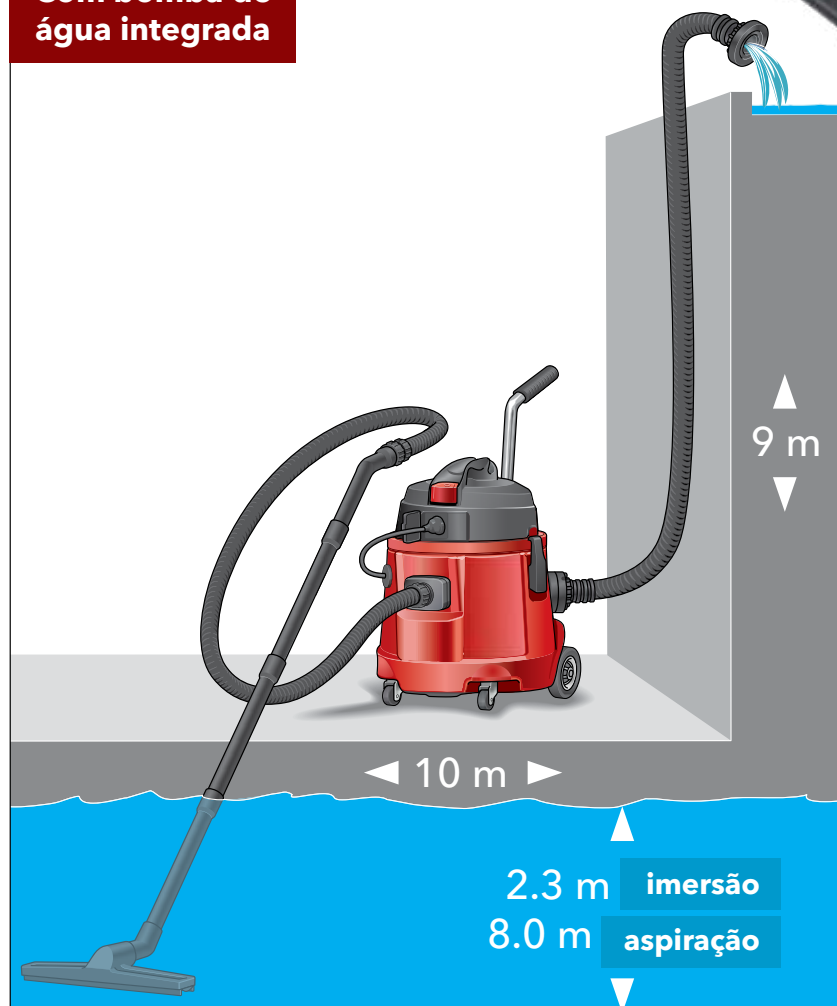
Mangueira para águas sujas de 10 m com ligação em C
